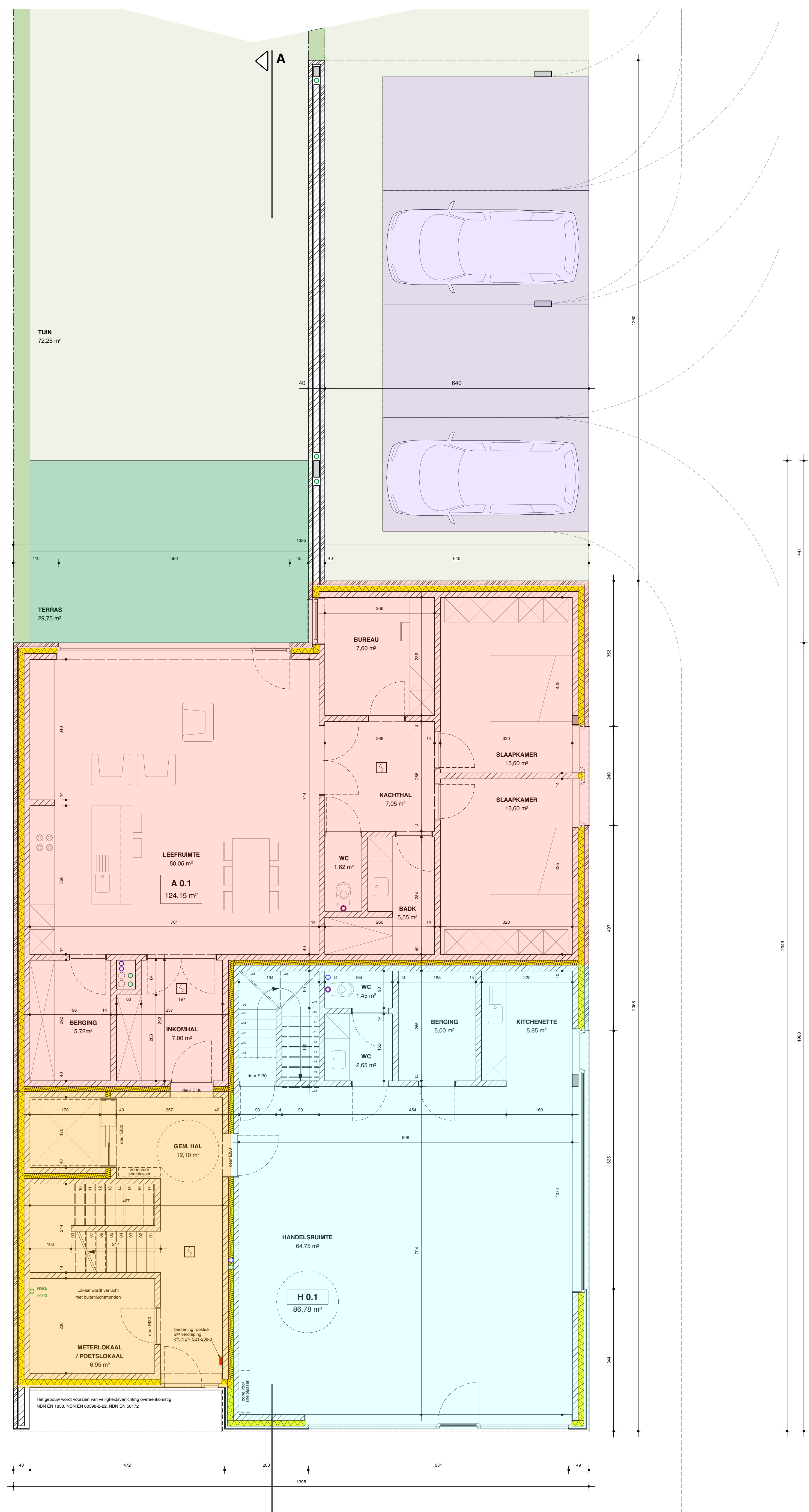
NIVEAU 0 schaal 1 : 50
