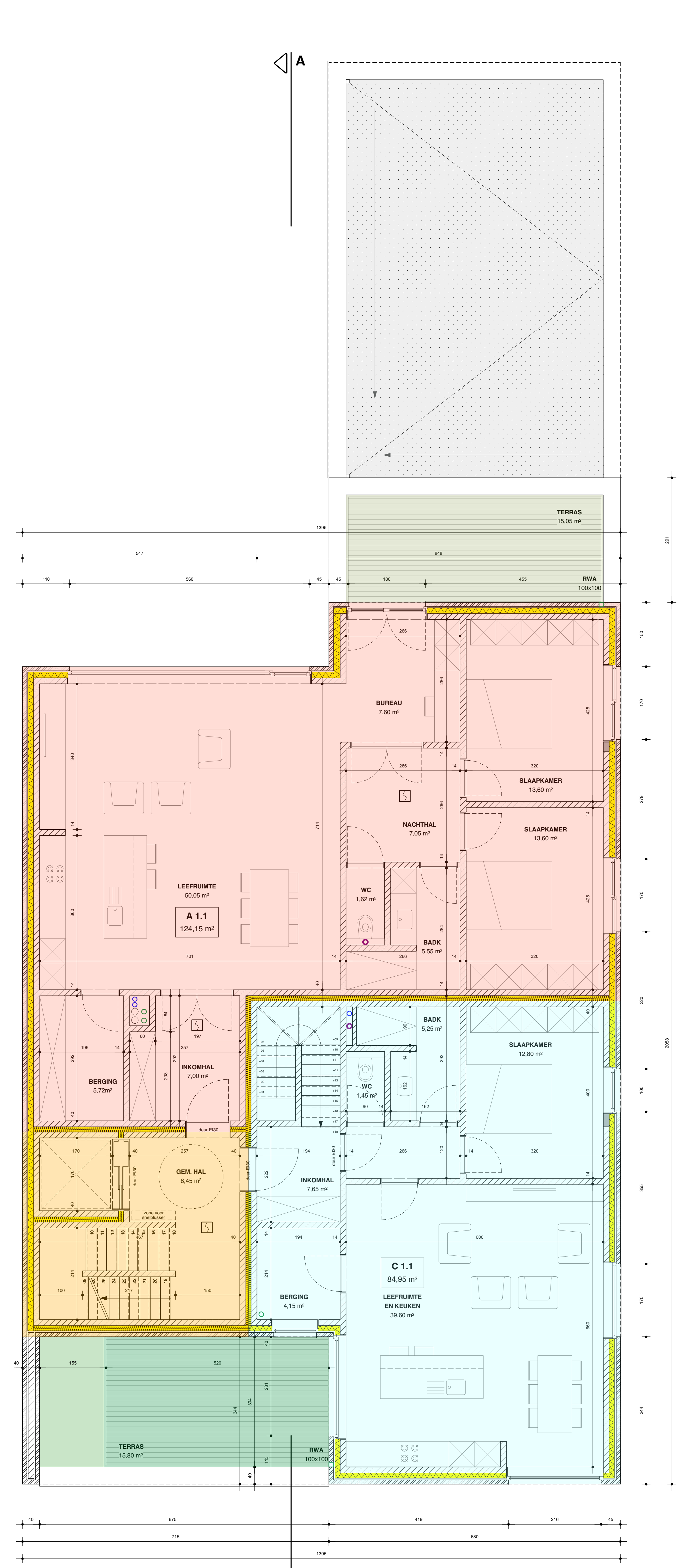
NIVEAU +1 schaal 1 : 50
